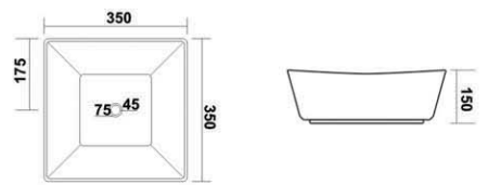
7017 - SLICE L 350, W 350, H 150mm
