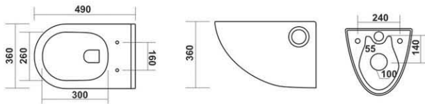
2010 - MOON L 490, W 360, H 360mm
