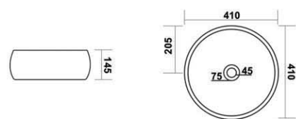
7004 - TITAN L 410, W 410, H 145mm
