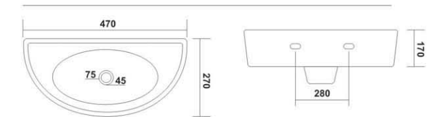
3009 - LIZA L 470, W 270, H 170mm
